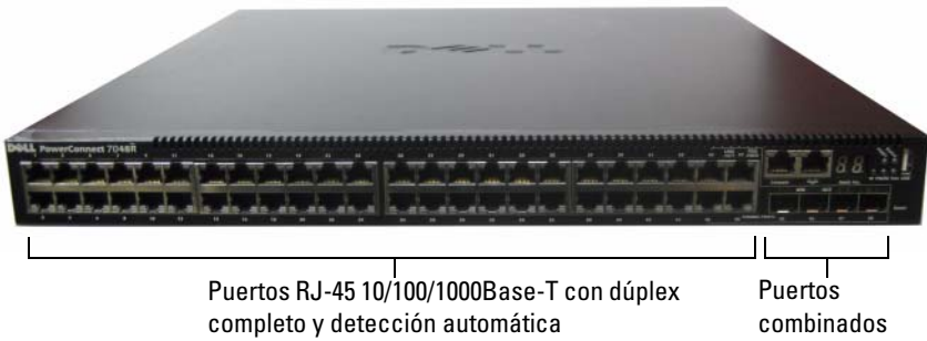
Ilustración 1-6. PowerConnect 7048R con 48 puertos 10/100/1000Base-T
