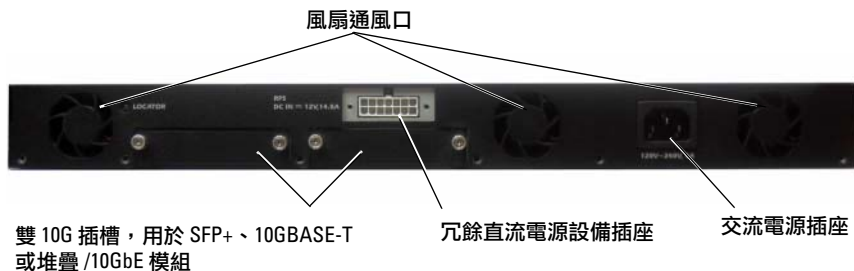
圖 1-9. PC7024P 和 PC7048P 背板
