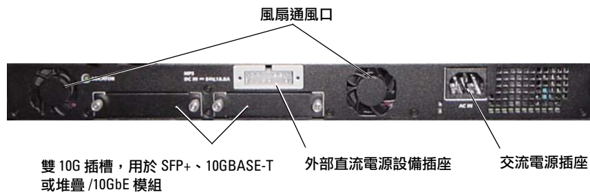
圖 1-10. PC7048R 背板
