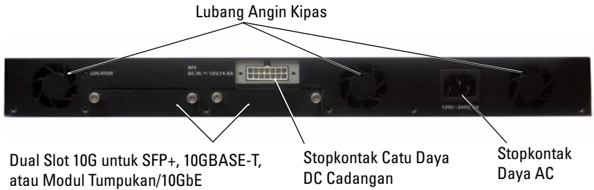
Gambar 1-9. Panel Belakang PC7024P dan PC7048P
